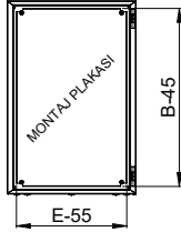
İÇ GÖRÜNÜŞ
